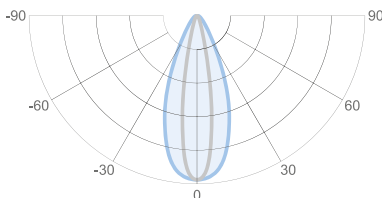
Диаграмма освещенности
