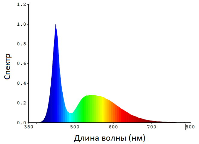
Спектрально-волновая диаграмма (Cool White)
