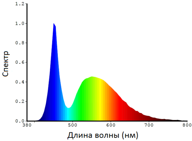
Спектрально-волновая диаграмма (White)
