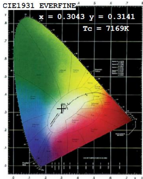
Диаграмма цветового пространства (White)
