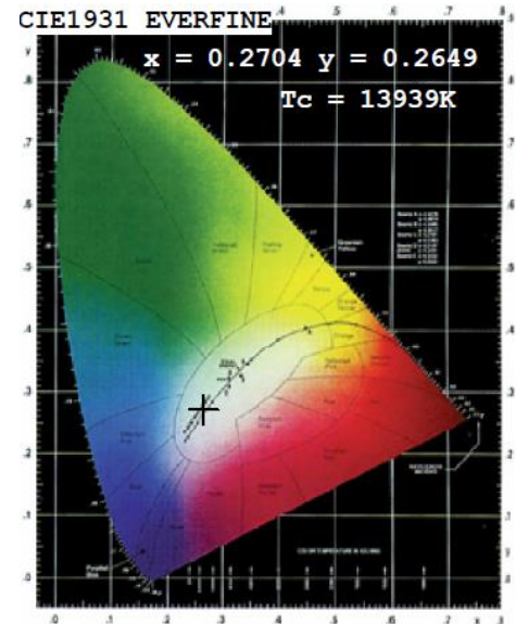
Диаграмма цветового пространства (Cool White)
